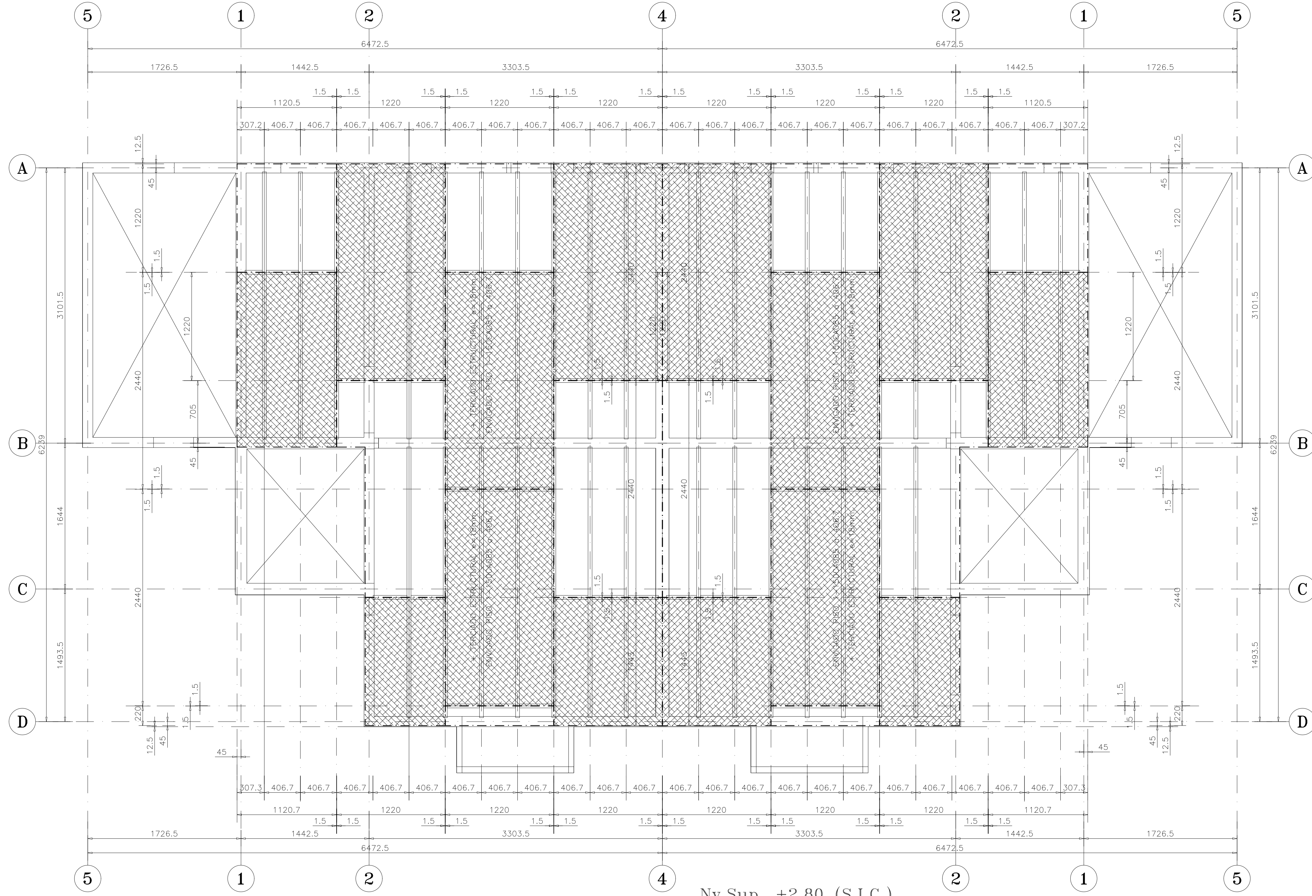
Nv.Sup. +2.80 (S.I.C.) PLANTA ENVIGADO DE PISO ESCALA 1:25
