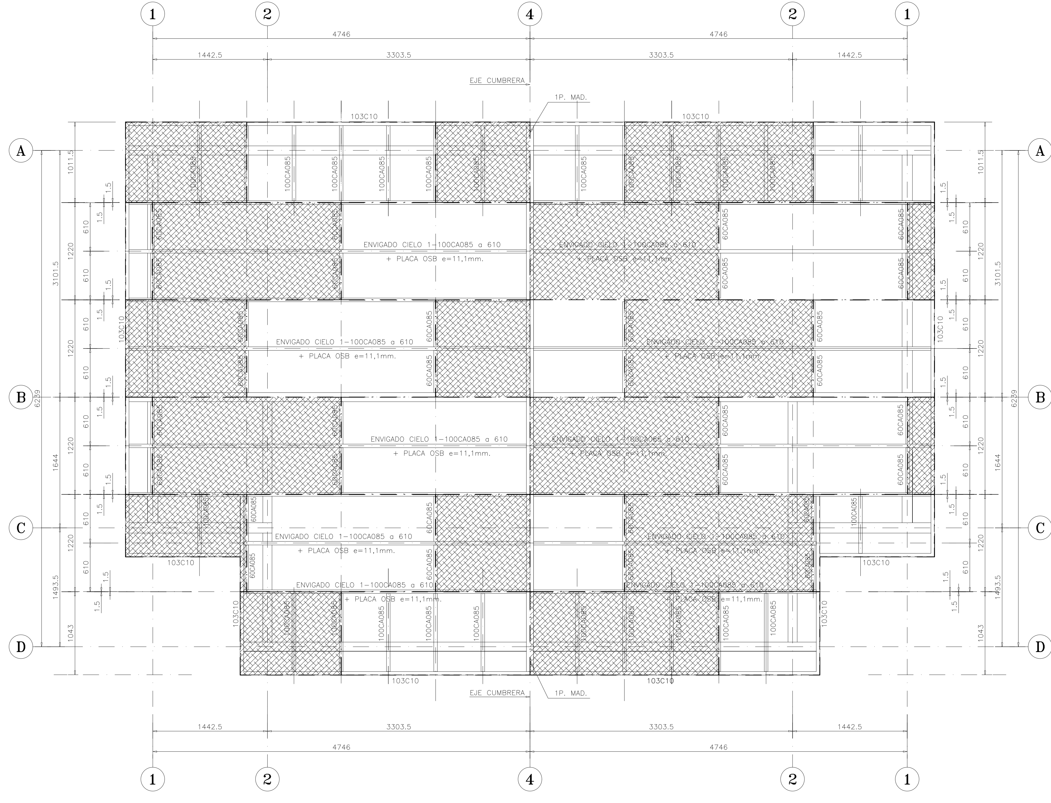
PLANTA ENVIGADO DE CUBIERTA ESCALA 1:25
