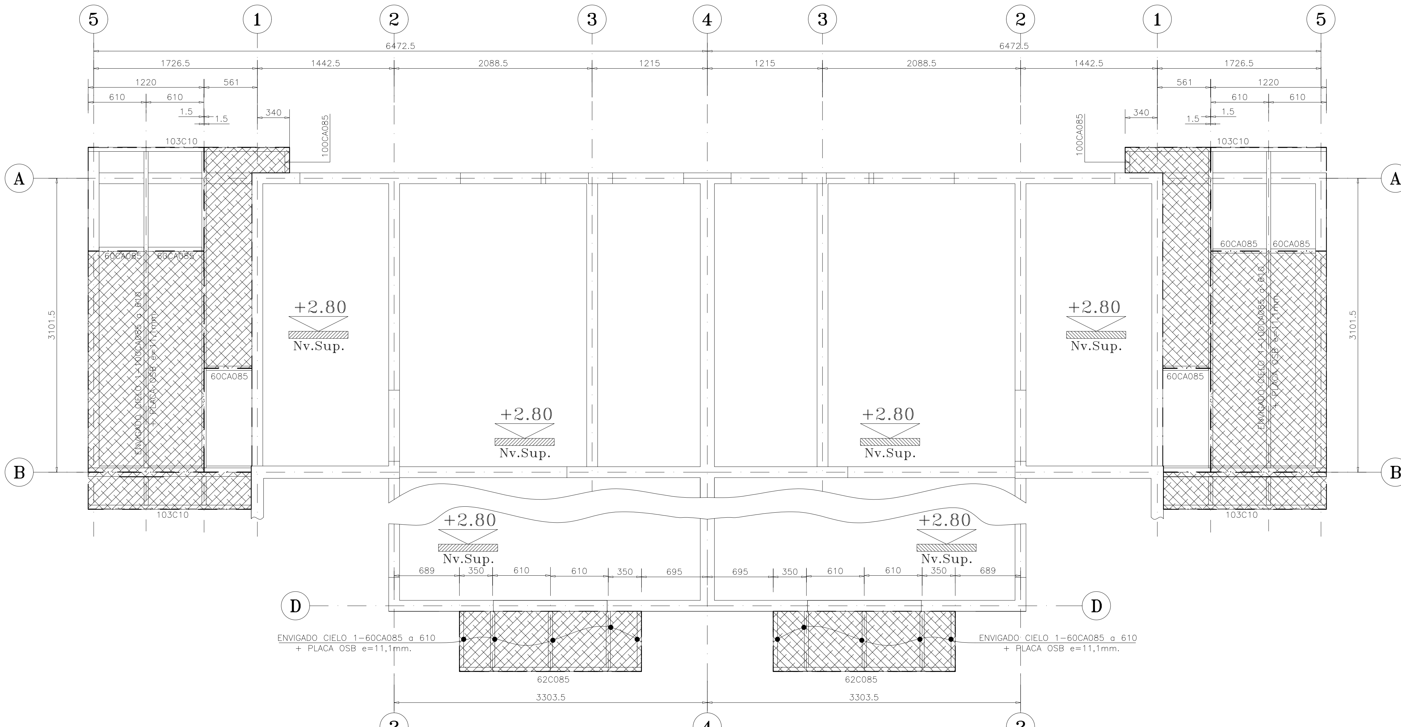
PLANTA ENVIGADO DE CUBIERTA 1ºPISO ESCALA 1:25
