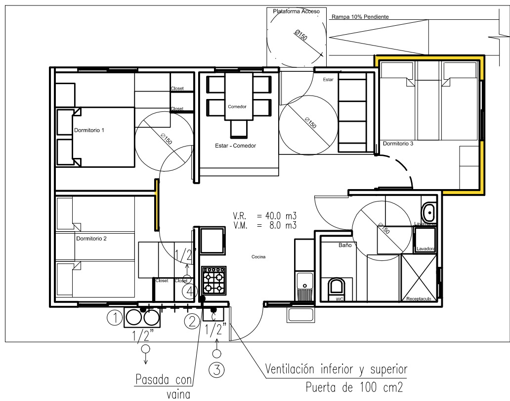
Casa Tipo E Planta Primer Piso ESCALA: 1/100
