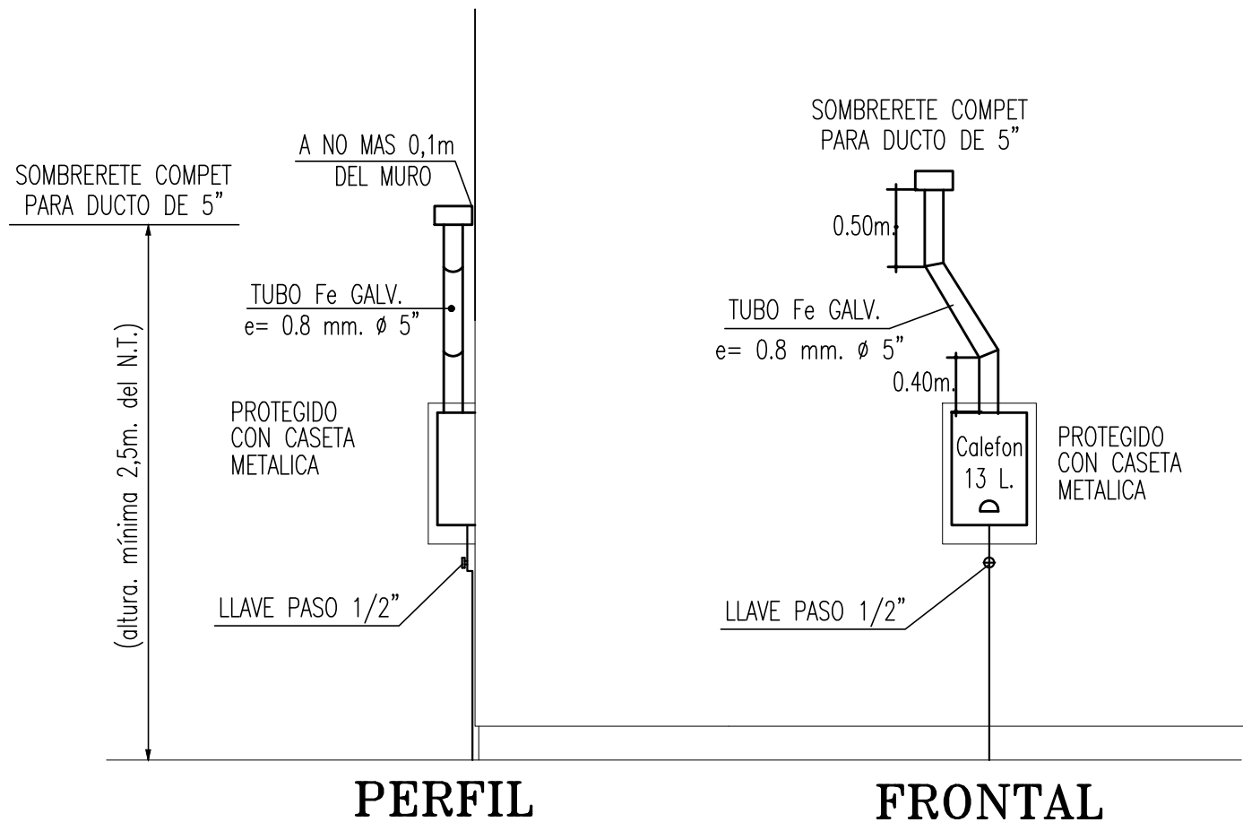
DETALLE CALEFON
