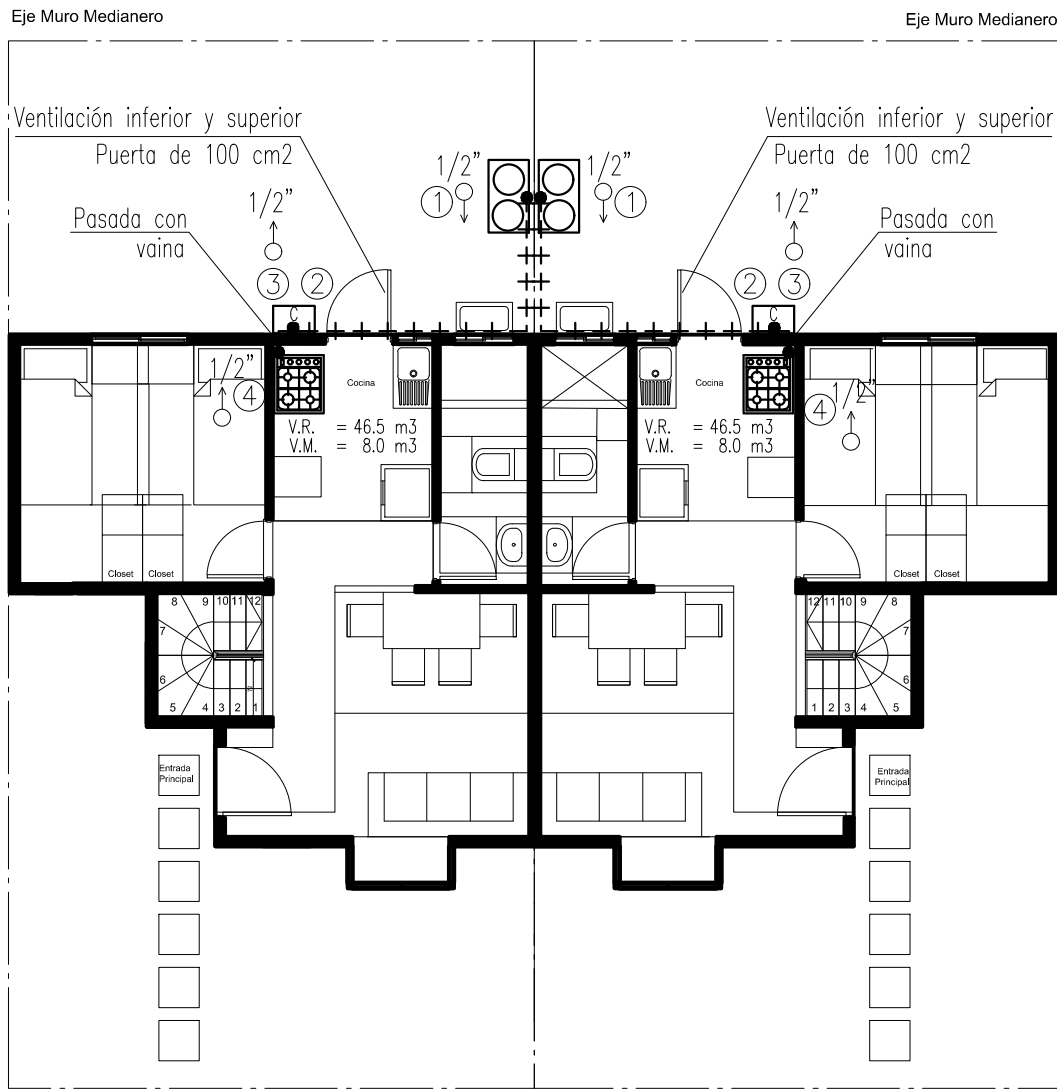
Casa Tipo B Planta Primer Piso ESCALA: 1/100
