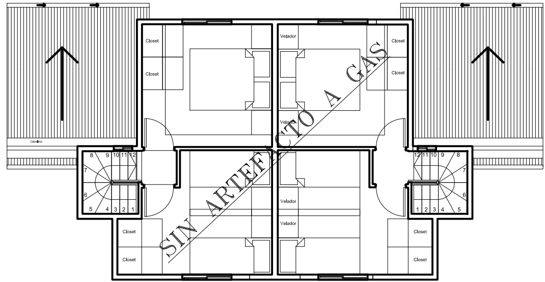
Casa Tipo B Planta Segundo Piso ESCALA: 1/100
