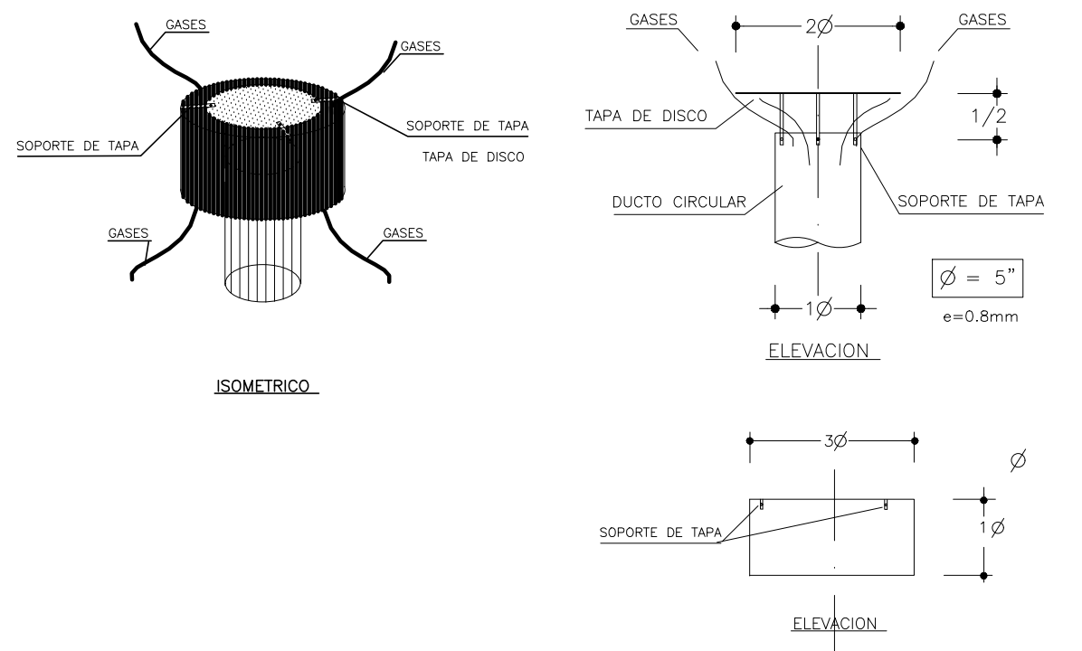
ESQUEMA SOMBRERETE TIPO COMPET (ART. 45 FIG. Nº45.1)
